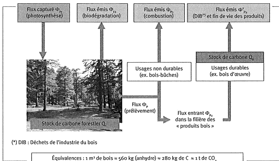
FIGURE 1 STOCKS ET FLUX DE CARBONE DANS LA FORÊT ET LES FILIÈRES D'UTILISATION DU BOIS
