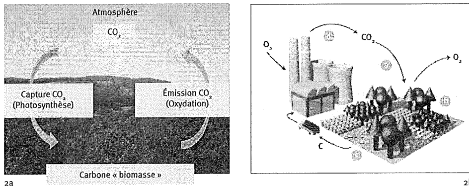
FIGURE 2 ILLUSTRATIONS DE LA NEUTRALITÉ CARBONE DE LA BIOMASSE
