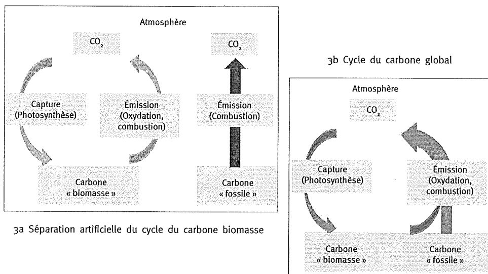
FIGURE 3 DEUX VISIONS DU CYCLE DU CARBONE TERRESTRE
